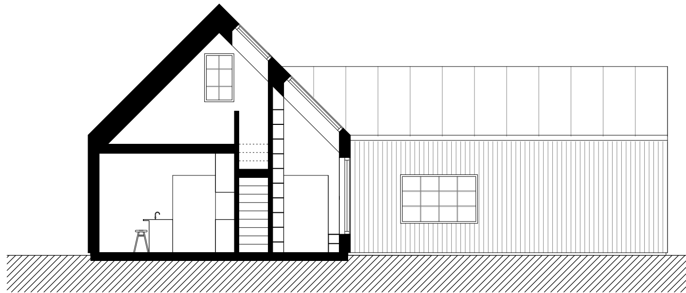
SEKTION KÖK
