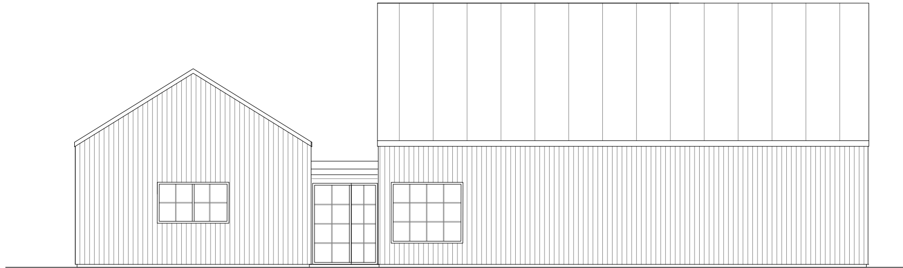
ENTRÈ
